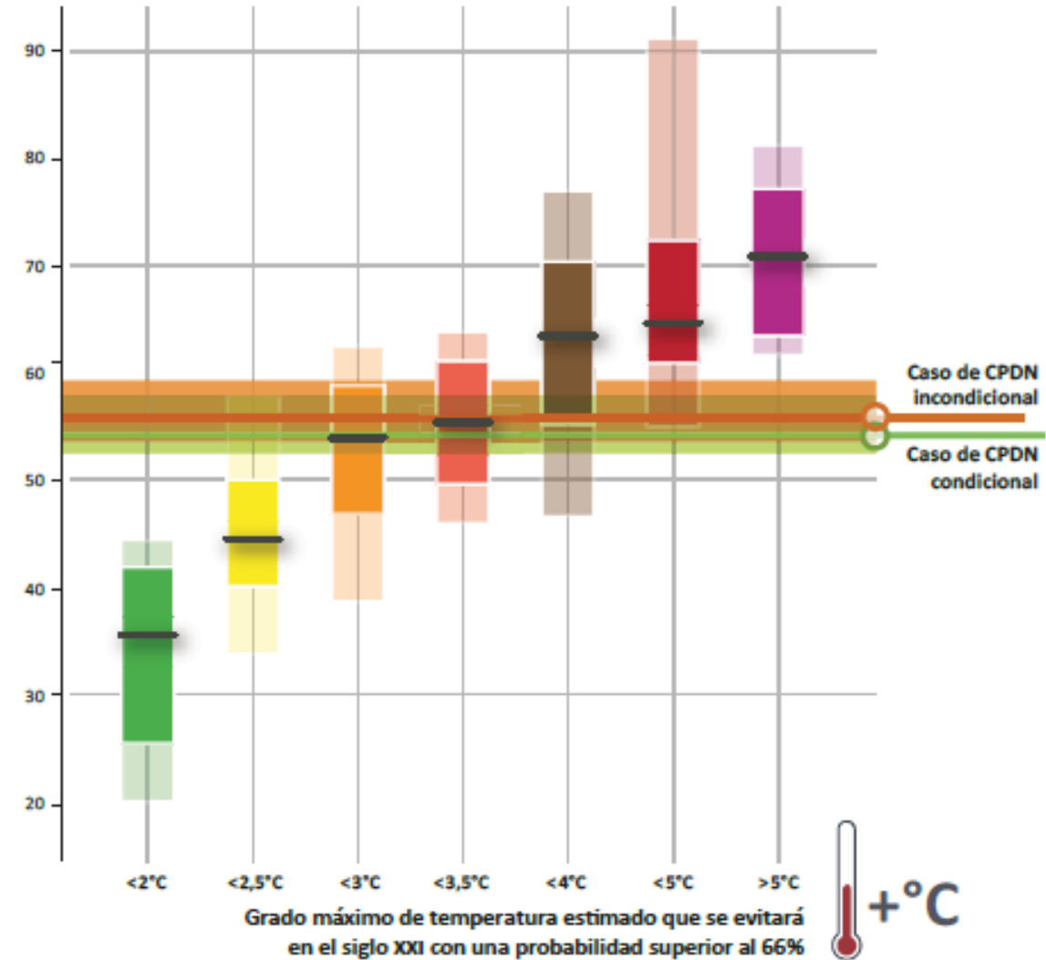
Niveles de emisión de GEI en 2030 (GtCO 2 e/año)
